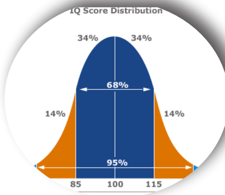
Statistiques I
